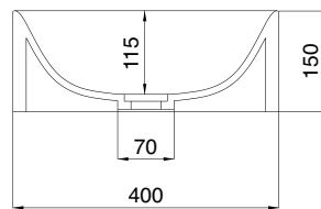
SEZIONE A-A
